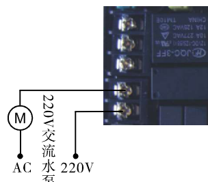
图3-7 进口接增压泵的接线图
