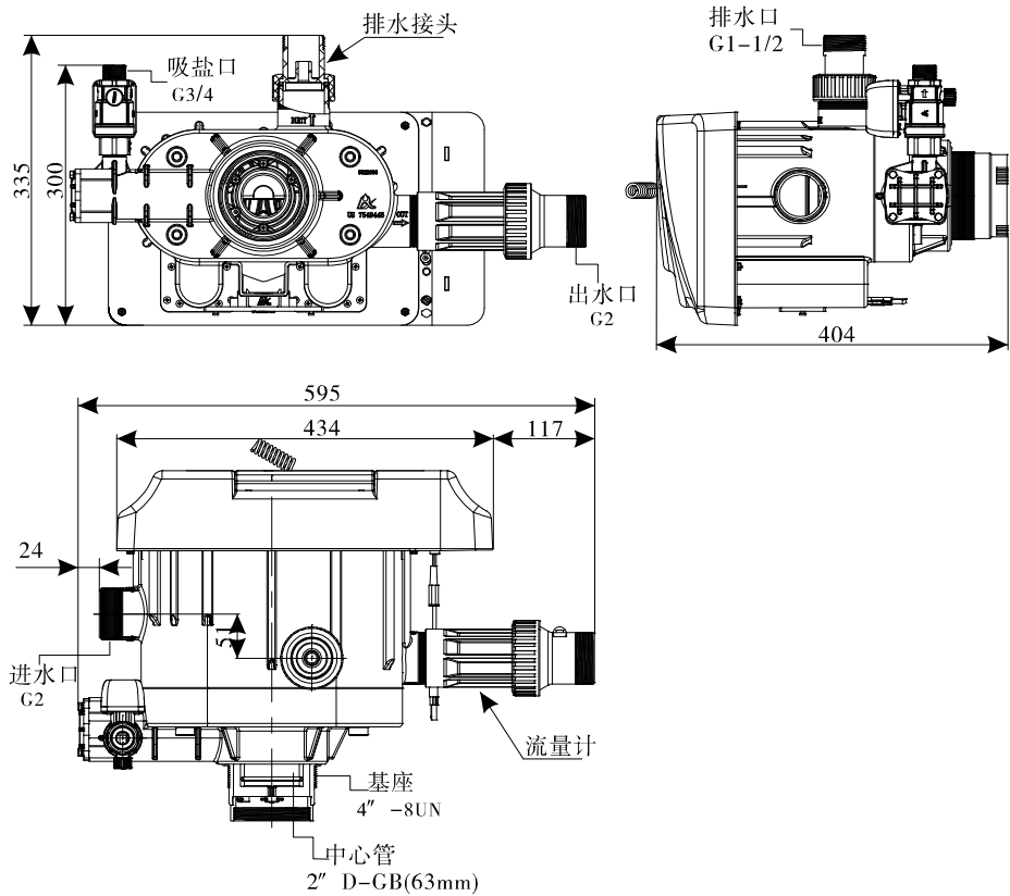
63620T结构图
