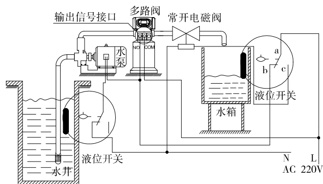
图3-5 通过水箱液位控制进水泵的接线图
