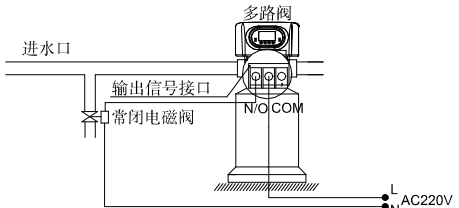
图3-3 泄压端口的接线图
