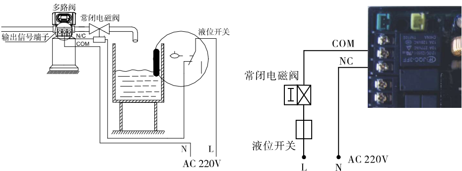
图3-1 控制出口电磁阀的接线图
