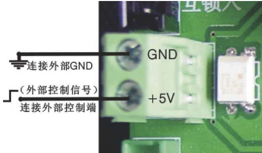
图3-11 远程控制端口的接线图
