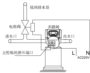
图3-10 泄压端口的接线图
