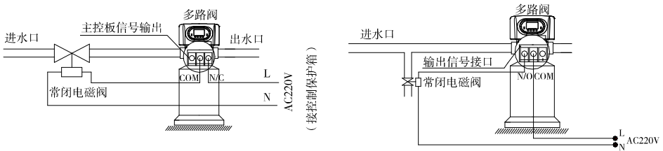
图3-3 控制进口电磁阀的接线图 图3-4 泄压端口的接线图
