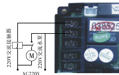
图3-9 进口接增压泵的接线图
