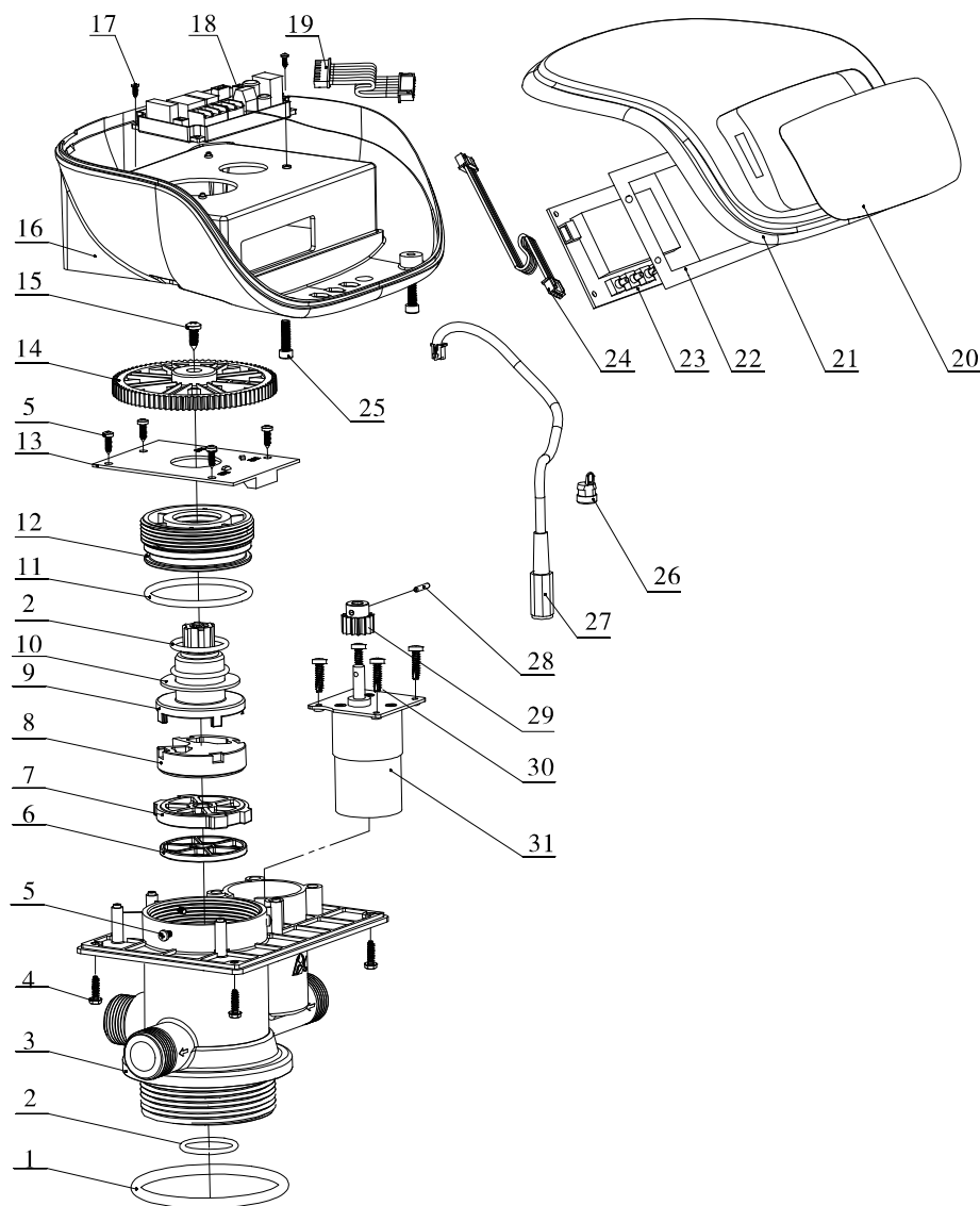
F71G1 (53502B) 结构图:
