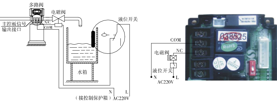
图3-2 控制出口电磁阀的接线图
