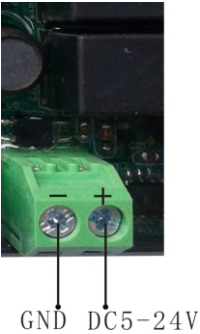
图3-9远程控制端口的接线图
