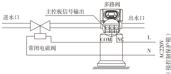
图3-2 控制进口电磁阀的接线图
