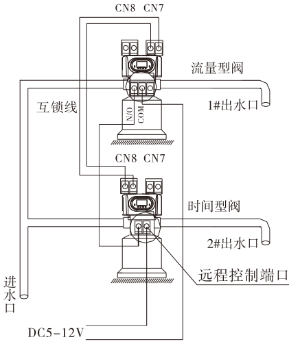
图3-10 同时供水，分别再生 图3-11 同时供水，顺序再生
