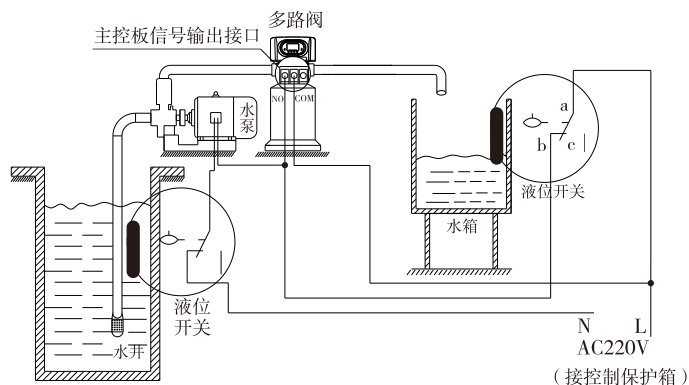
图3-4 通过水箱液位控制进水泵的接线图
