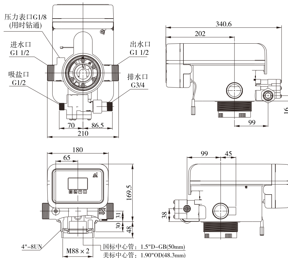
63508/63608结构图
