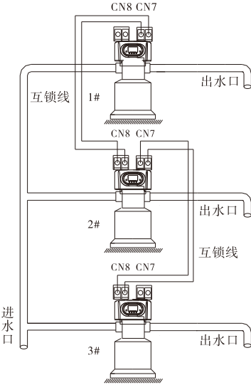
图3-10 同时供水，分别再生 图3-11 同时供水，顺序再生
