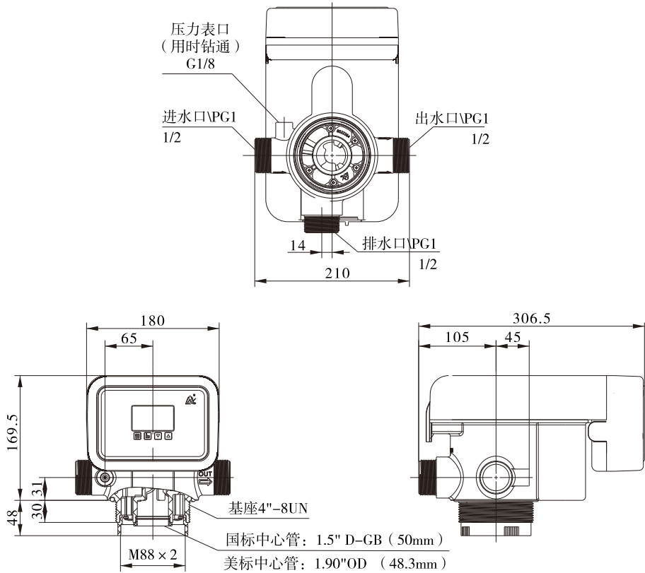
53508/53608结构图
