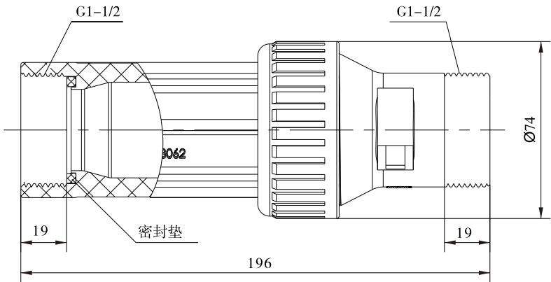
5447010流量计结构图
