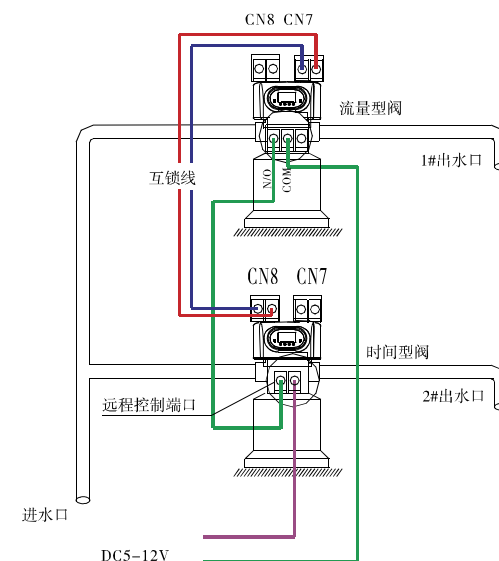
图 3-13 同时供水，顺序再生
