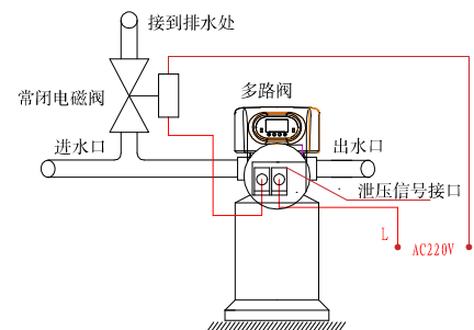
图 3-10 泄压端口的接线图
