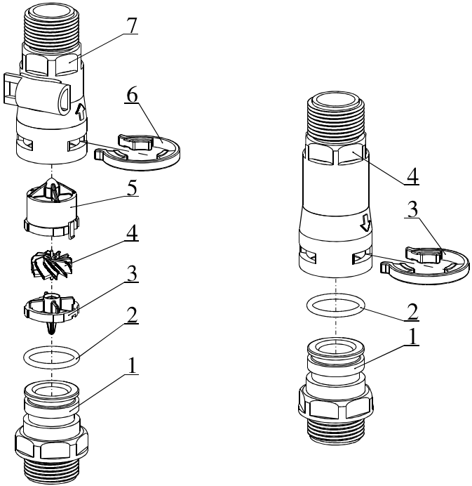
5447020流量计
