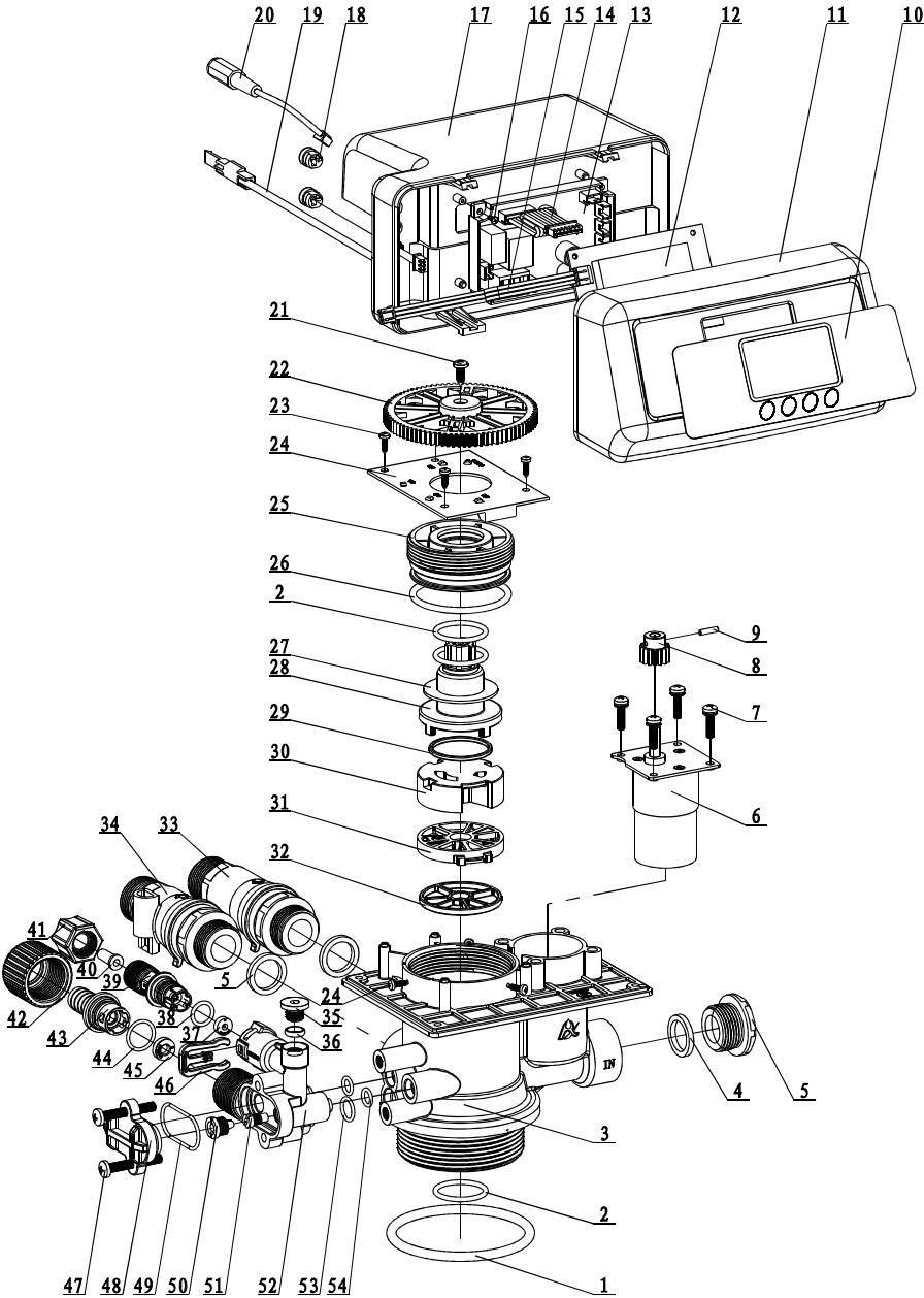
F117A3的结构图
