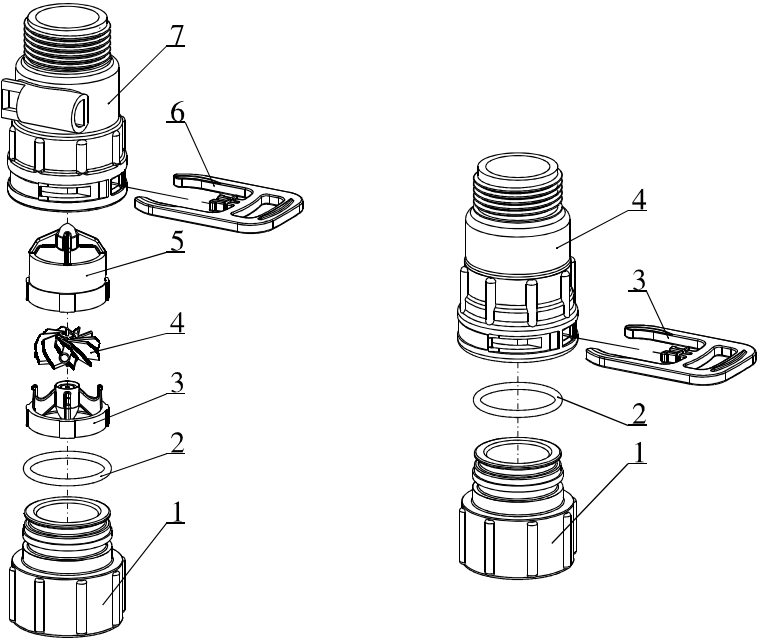
5447018流量计
