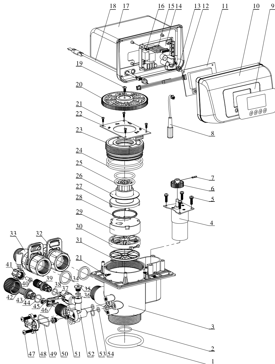
F116A3的结构图
