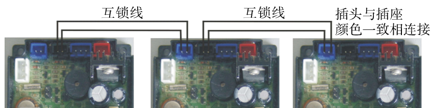
图 3-9 互锁的接线图
